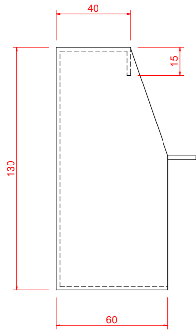
aanzicht voorzijde
