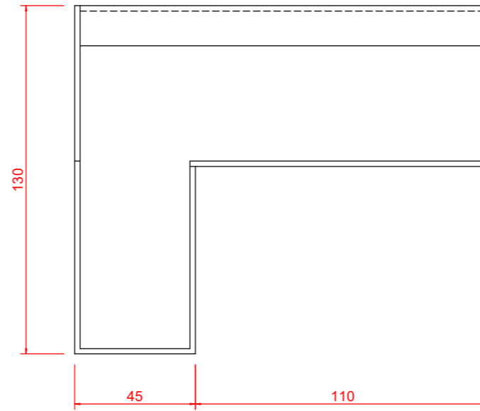
aanzicht binnenzijde
