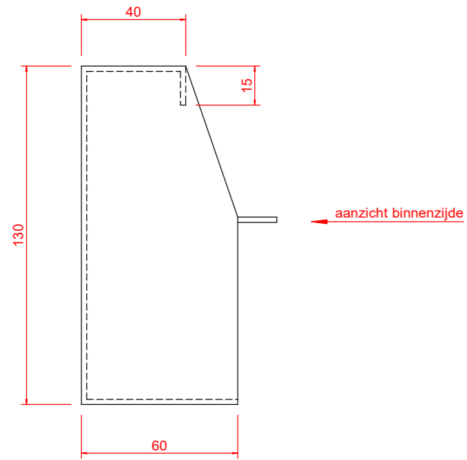
aanzicht voorzijde
